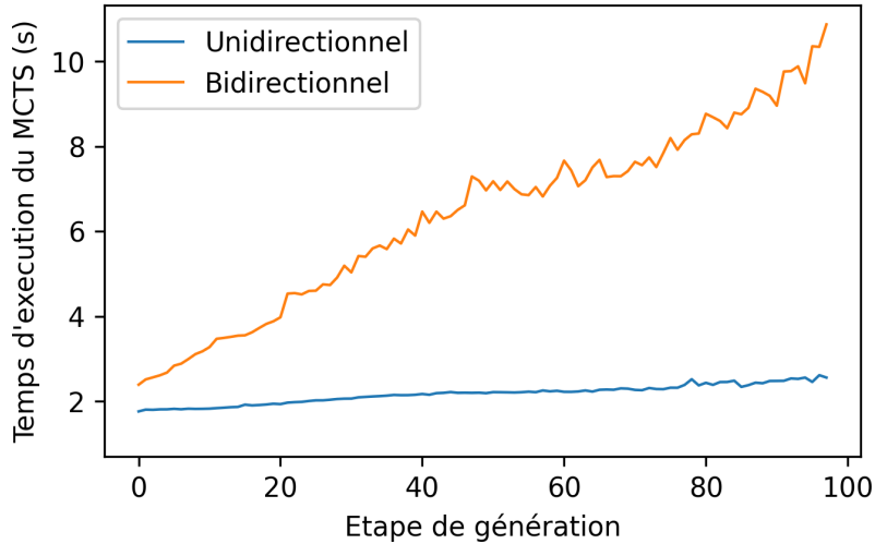
FIGURE 7 – Temps d’exécution des itérations MCTS (s) en fonction du nombre d’étapes de génération (moyenné sur 10 batchs de 30 séquences ; amazon_polarity)
