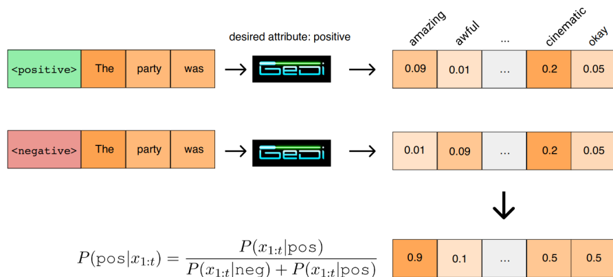
FIGURE 2 – Schéma illustrant le principe de classification de GeDi sur un problème de classification à 2 classes ( positive vs. negative ), tiré de (Krause et al. , 2021). En 2 passes, l’une avec le token de contrôle de la classe positive et l’autre avec le token de la classe négative, on obtient un score pour chacun des token du vocabulaire.
