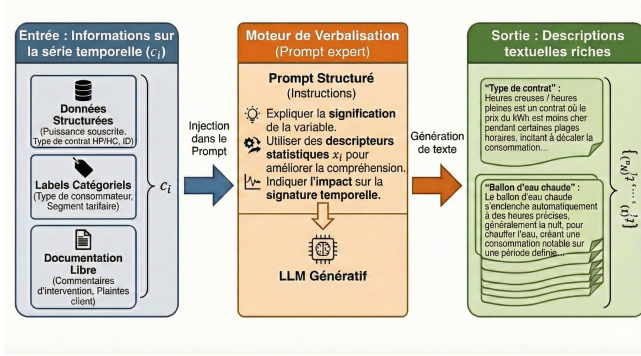
(a) Pipeline de verbalisation.
