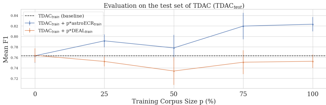
FIGURE 3 – Evaluation sur \text{TDAC}_{\text{test}} d'un système de détection d'entités nommées à base d'un modèle astroBERT pour la détection d'entités nommées en fonction de la taille du corpus d'entraînement.
