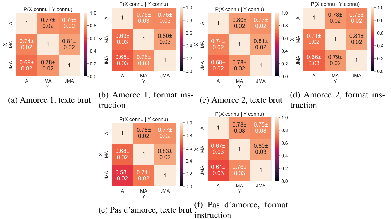
FIGURE 9 – Effet de l'ajout d'explications sur les concepts temporels par le biais d'une amorce explicative (cf. Annexe C.3)
