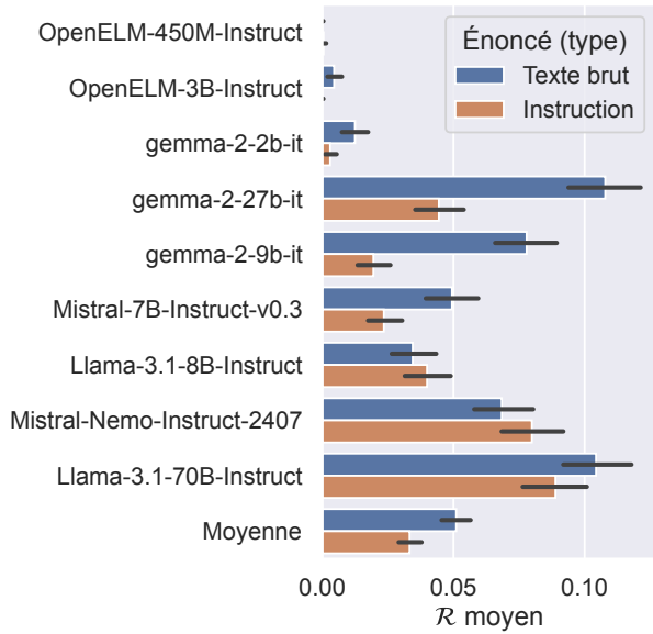
FIGURE 4 – Moyenne de \mathcal{R} sur toutes les granularités des faits de TimeStress suivant le format des énoncés soumis aux modèles : texte brut (bleu) ou instruction (orange). Les intervalles de confiance à 95% (bootstrap) sont affichés.
