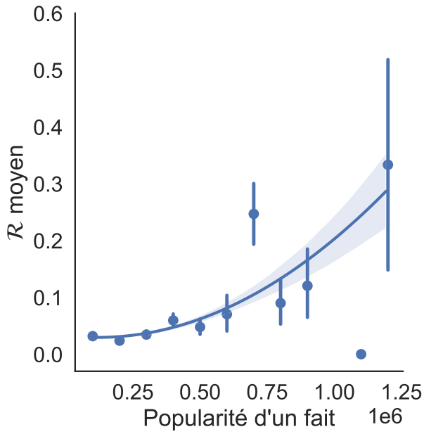
FIGURE 12 – Relation entre la popularité des faits et la métrique de robustesse calculée sur l'ensemble des ML et des granularités A, MA et JMA.
