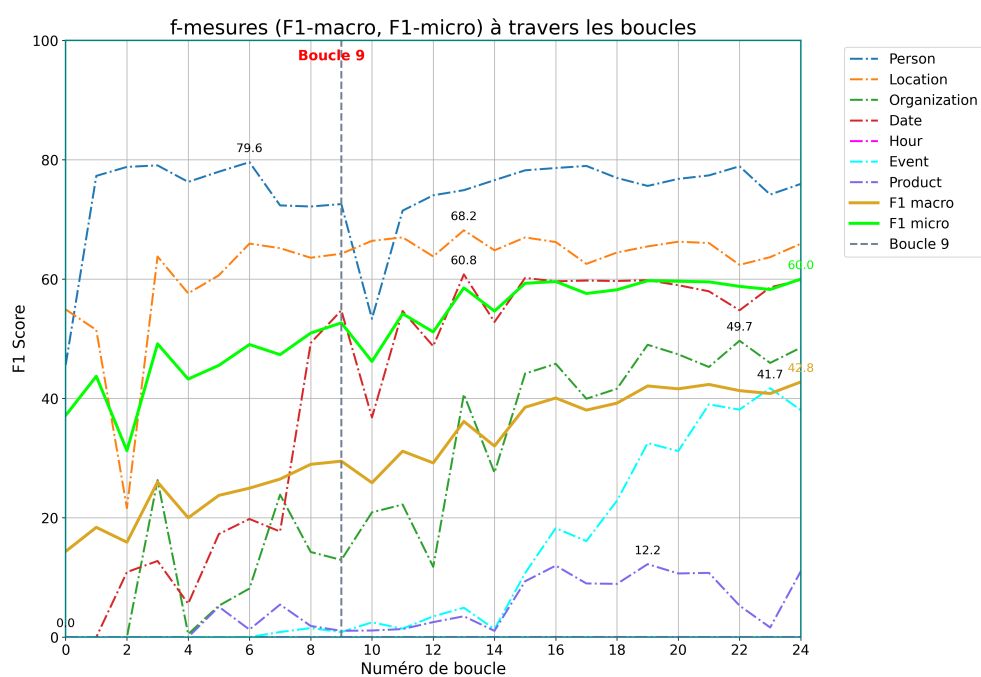
FIGURE 4 – Apprentissage actif sur 24 boucles - avec optimisation des hyper-paramètres
