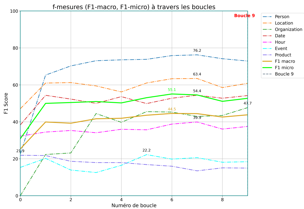
FIGURE 3 – Apprentissage actif - avec augmentation des données
