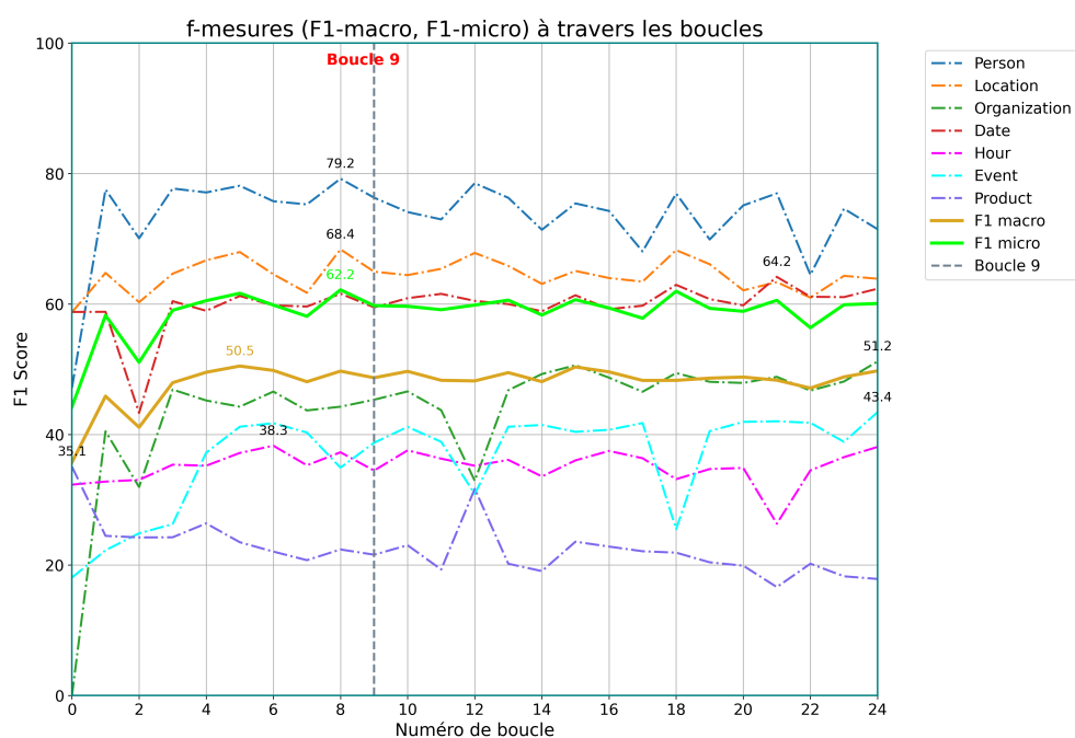
FIGURE 5 – Apprentissage actif sur 24 boucles - avec augmentation des données et optimisation des hyper-paramètres
