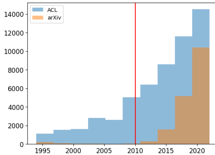
FIGURE 7 – Histogrammes du nombre d'articles issus de l'Anthologie ACL et d'ArXiv par année, sur la période commune 1952-2022. Les distributions sont davantage similaires entre 2010 et 2022 qu'avant, ce qui permet la comparaison des structures de résumés sur cette période par des diagrammes de Sankey.
