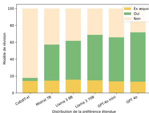
FIGURE 2 – Distribution de la préférence étendue humaine pour chaque modèle de révision. La zone verte correspond aux cas où le modèle est préféré.
