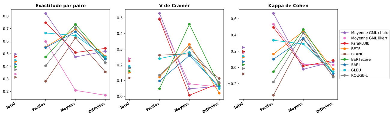
FIGURE 6 – Alignement des métriques automatiques avec les annotations humaines, par difficulté. Les triangles de la première colonne représentent l’accord sur l’ensemble des données de la Table 4
