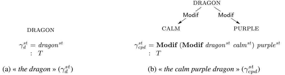
FIGURE 6 – Représentation de SSyntS associées aux expressions nominales « the dragon », « the calm purple dragon » et des termes objets (de \Lambda(\Sigma_{st}) ) associés.
