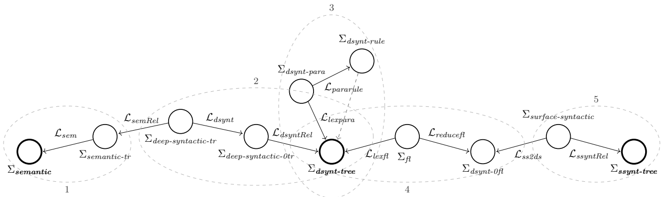
FIGURE 4 – Composition des ACG de l'implémentation de MTT
