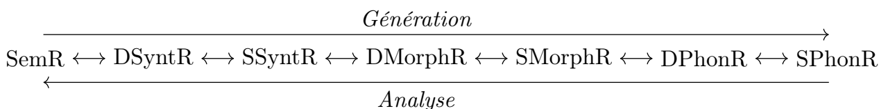
FIGURE 1 – Schéma du modèle sens-texte ( Mel’čuk et al., 2012 )
