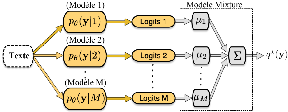
FIGURE 1 – Notre mélange, les poids \{\mu_i\} sont associés à chaque token et à chaque modèle.
