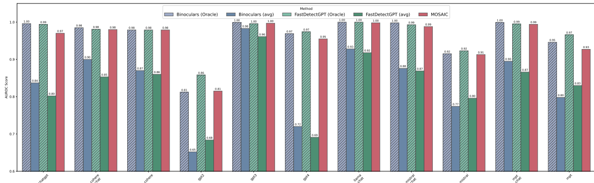
FIGURE 2 – Comparaison des AUROC de MOSAIC sur le jeu de données RAID avec les modèles Llama et Tower. Les noms des modèles représentent le modèle utilisé pour générer le jeu de données.
