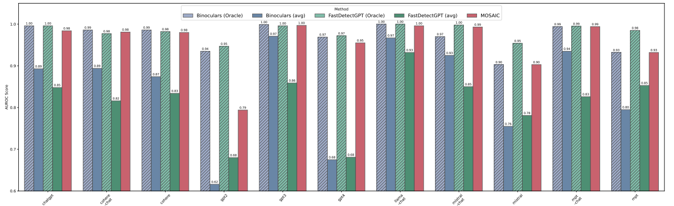
FIGURE 3 – Comparaison des AUROC de MOSAIC sur le jeu de données RAID avec les modèles Falcon. Les noms des modèles représentent le modèle utilisé pour générer le jeu de données.
