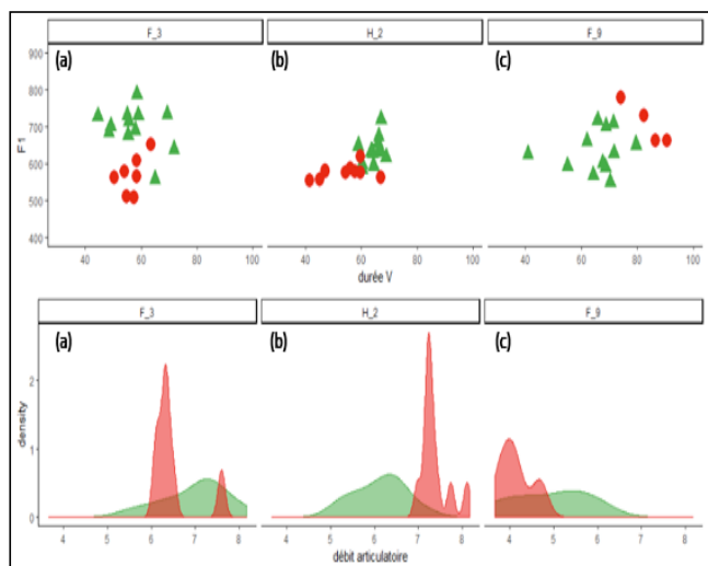
FIG.4 – Illustration sur trois locuteurs types (H_3, H_2 et F_9) des profils de modifications entre les tâches RepetConfo (rouge) et Lecture (vert). La relation entre F1 et durée de la voyelle /a/ est présentée en haut, et la distribution du débit selon les phrases en bas.
