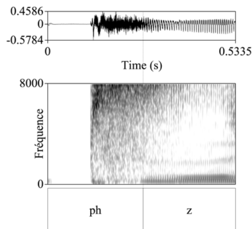
FIGURE 4 : Le signal acoustique et le spectrogramme de la forme /p h zɹ/, produite par FS1.
