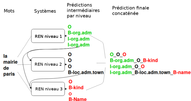
FIGURE 2 – Représentation de notre implémentation en 3 étapes
