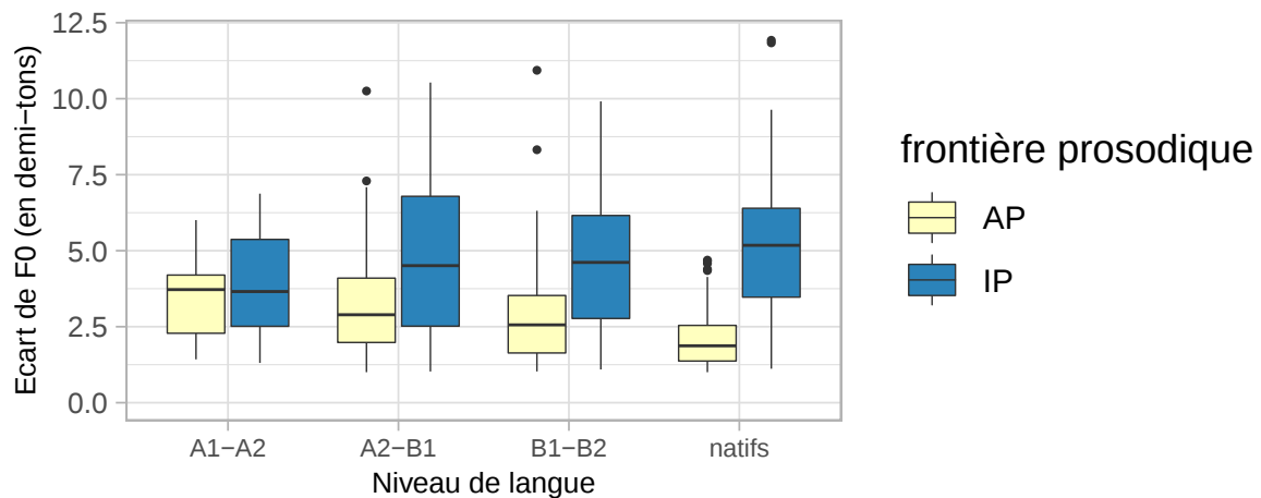
FIGURE 2 – Ecart de F0 (en demi-tons) selon la frontière prosodique et le niveau de langue
