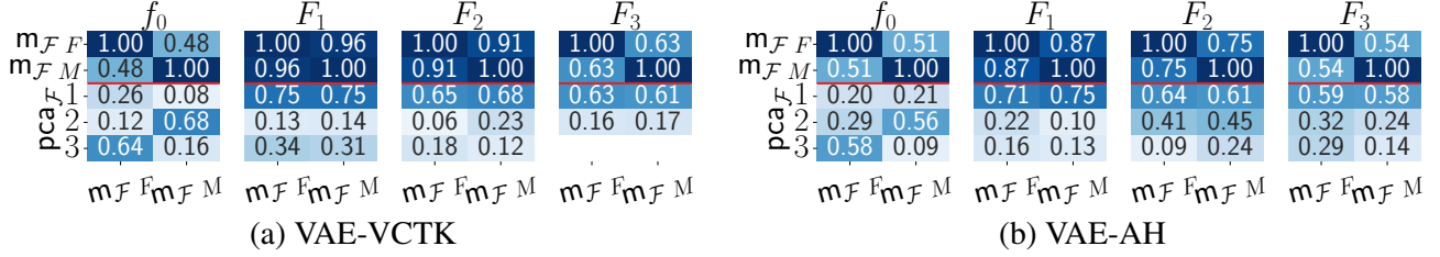
FIGURE 2 – Similarité cosinus entre m_{F|M} , m_{F|F} et pca_F . Pour plus de clarté, seules les trois premières composantes principales sont présentées.
