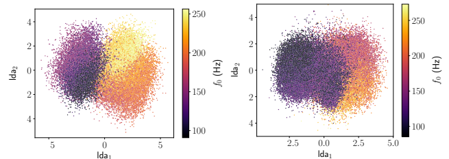
FIGURE 4 – Projection de NS_z^{VCTK} (gauche) et NS_z^{AH} (droite) sur les deux premières composantes de leurs lda respectifs, colorés en fonction de leurs valeurs f_0 .
