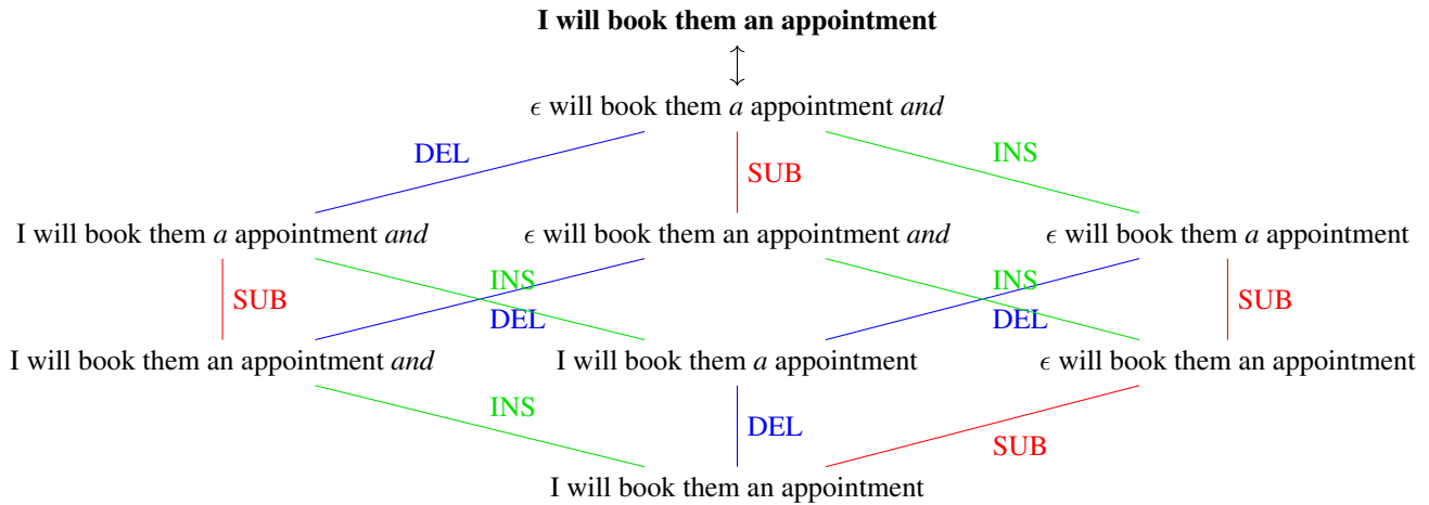
FIGURE 1 – Graphe de chaque modification possible pour obtenir une hypothèse sans erreur avec le paradigme minWED. Chaque arête correspond à une erreur corrigée. Étant donné la référence, nous avons trois erreurs de mots, chacune d'un type différent : 1 substitution, 1 insertion, 1 suppression. La métrique est basée sur la règle "le plus faible le meilleur". Le symbole \epsilon correspond à une suppression.
