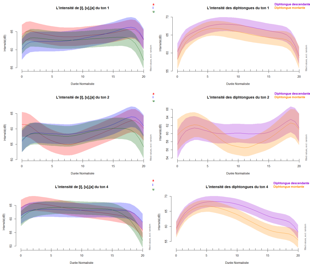
FIGURE 2 – Les courbes d’intensité prédites par les modèles de GAMMs pour les monophthongues [i], [u], [a] (à gauche), les diphtongues montantes[ia], [ua] et diphtongues descendantes [ai], [au] (à droite) pour chaque ton. L’intensité est représentée en y.
