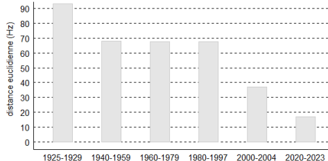
FIGURE 4 : Distances euclidiennes entre moyennes (Hz) entre /a/ et /ɑ/ en position finale de mot, formule : d = \sqrt{((F2\_a - F2\_ɑ)^2 + (F1\_a - F1\_ɑ)^2)} .
