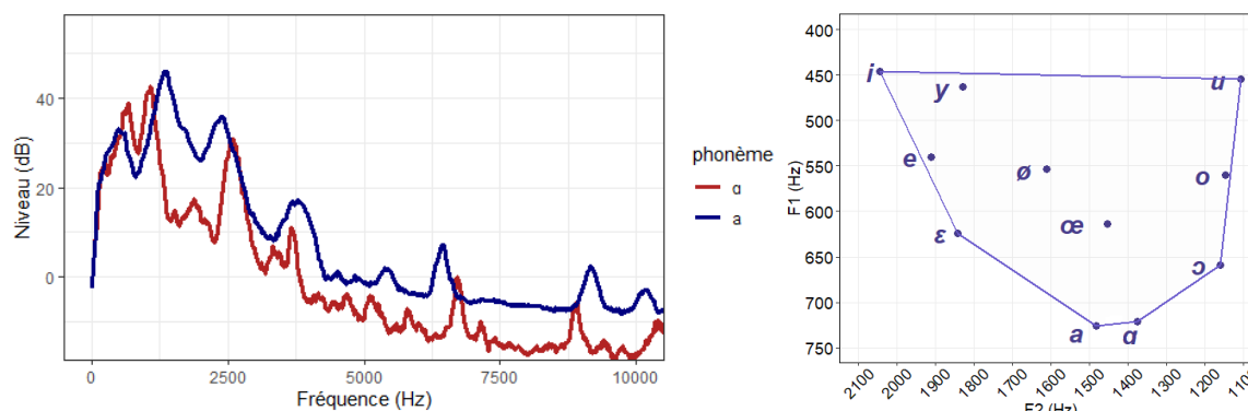
FIGURE 1 : À gauche : spectres comparés de /ɑ/ ( place ) et /a/ ( passe ) ; à droite : trapèze des voyelles orales (F1 et F2 en Hz) produites par un locuteur masculin, archives BnF, 1927.
