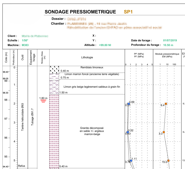
FIGURE 1 – Coupe de sondage tronquée, montrant 4 couches de lithologie (e.g. “ remblais limoneux ” entre 0 et 0,4 mètres de profondeur), une échelle de profondeur sur la gauche, et un identifiant ( SP1 ).
